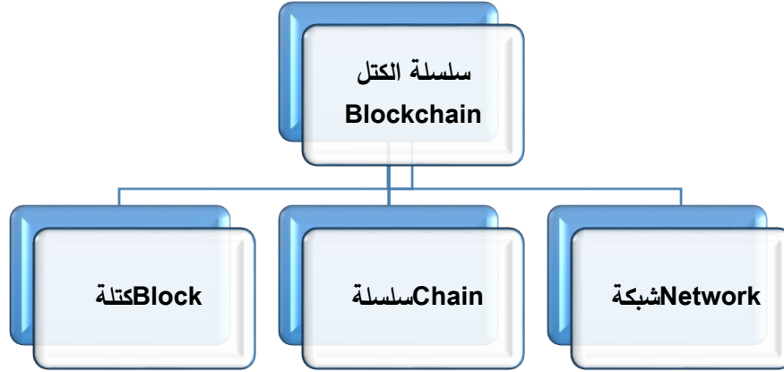
هيكل البلوكتشين (1)
